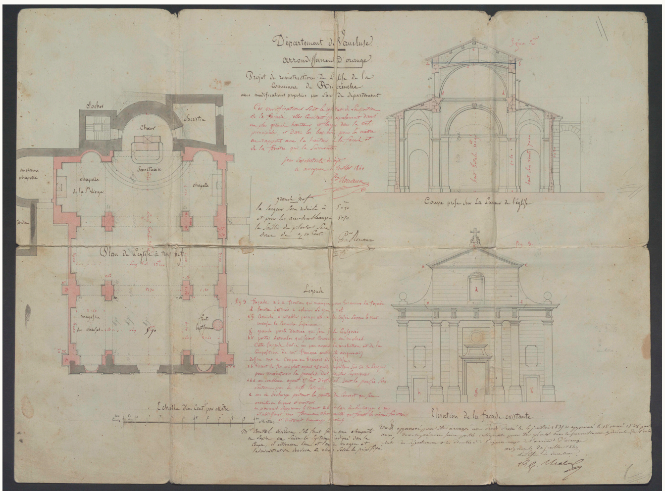
Plan projet reconstitution église - Juillet 1840
