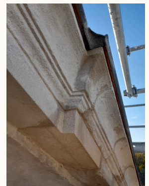
Photos 3 et 4 Remplacement des pierres les plus dégradées
